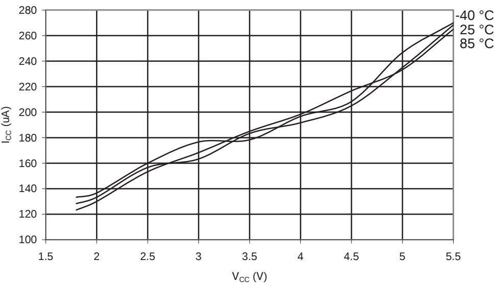
Figure 27-40. ATmega1284P: ADC Current vs. V CC (AREF = AV CC )
